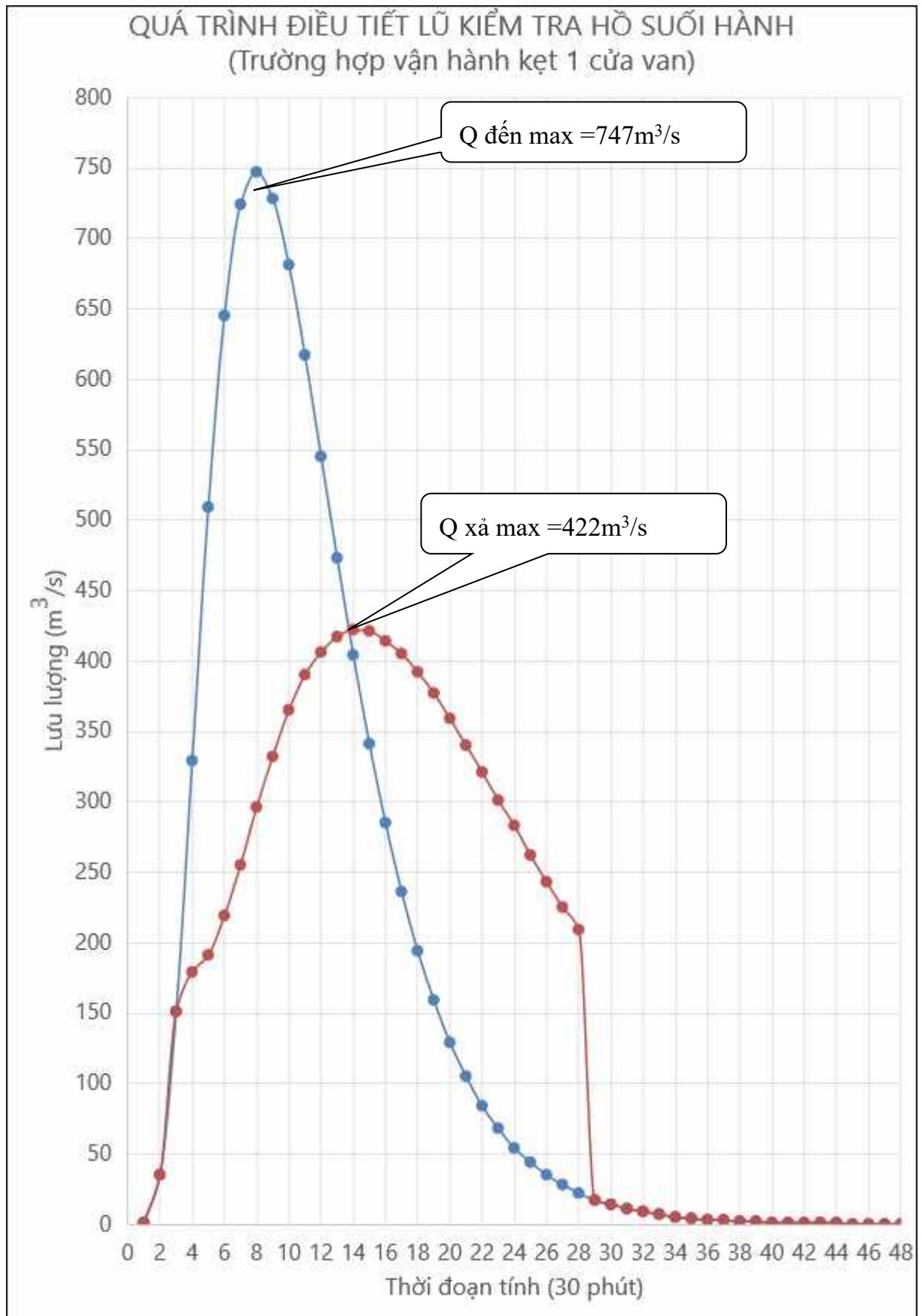
Hình PL 4.4: Quá trình điều tiết lũ kiểm tra – trường hợp kệt 1 cửa van
