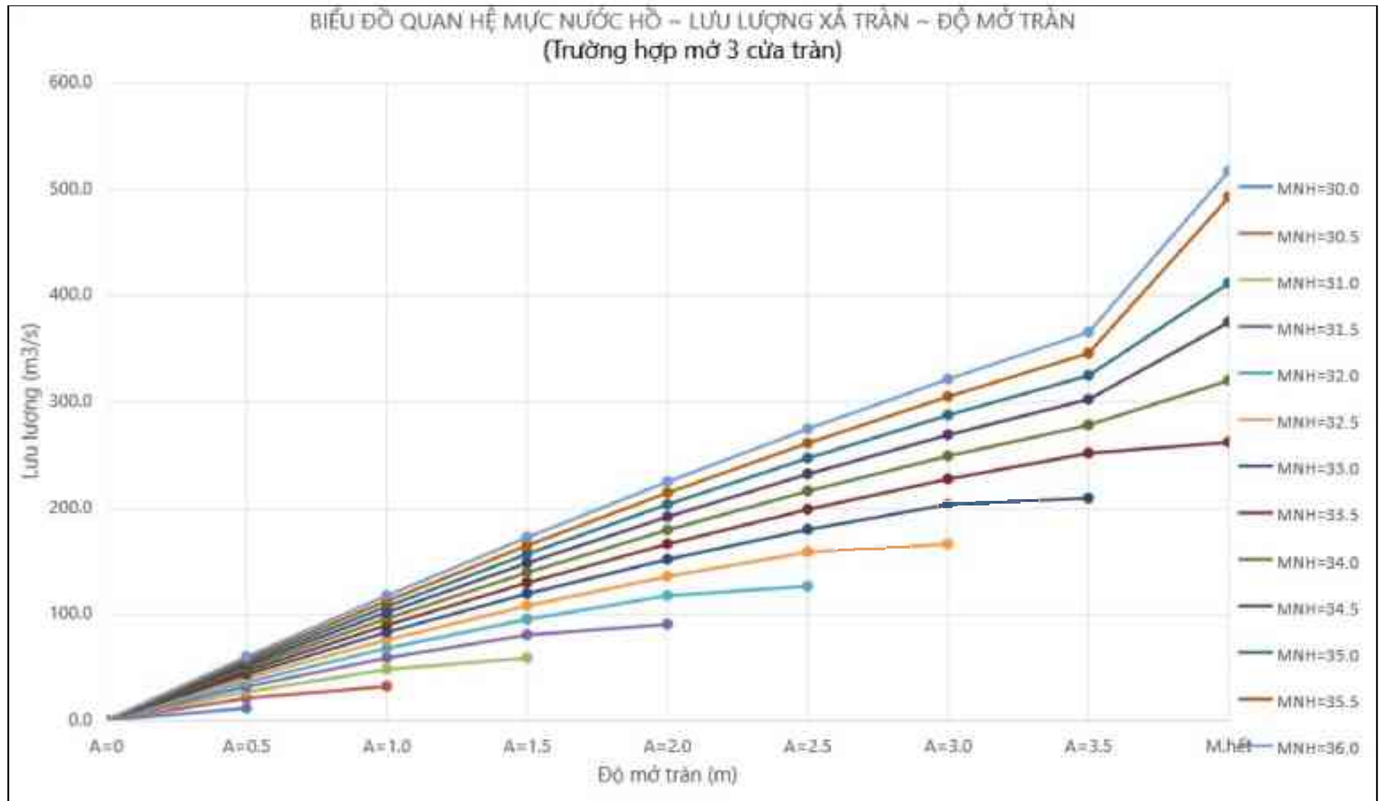
Hình PL 5.3: Lưu lượng qua tràn ~ Mức nước hồ ~ Độ mở cửa van (Trường hợp mở 3 cửa)
