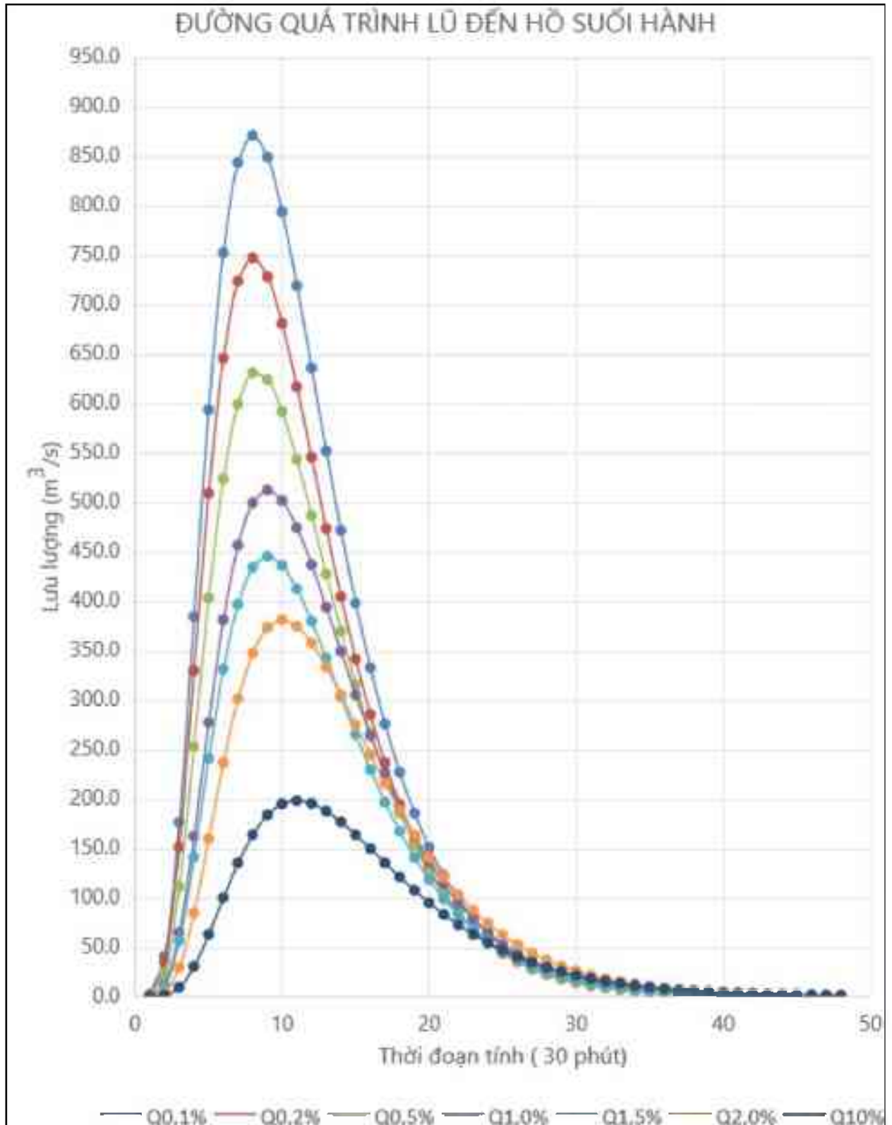
Hình PL 2.2 : Hình vẽ quá trình lũ đến hồ Suối Hành
