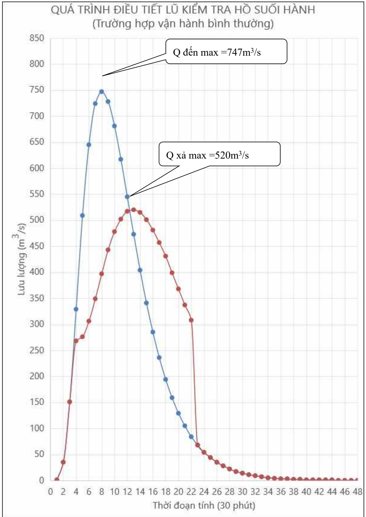
Hình PL 4.3: Quá trình điều tiết lũ kiểm tra hồ Suối Hành
