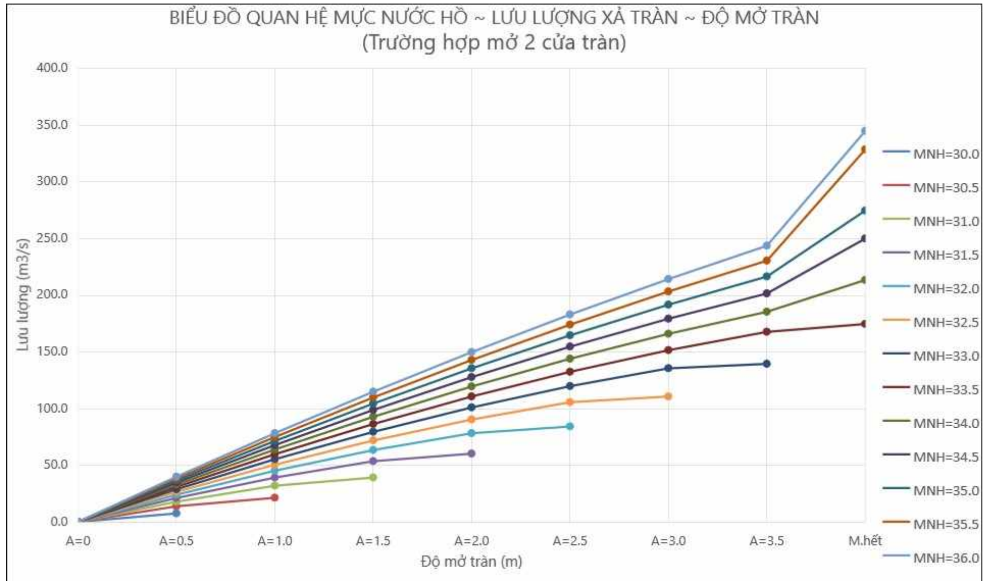
Hình PL 5.2: Lưu lượng qua tràn ~ Mức nước hồ ~ Độ mở cửa van (Trường hợp mở 2 cửa)
