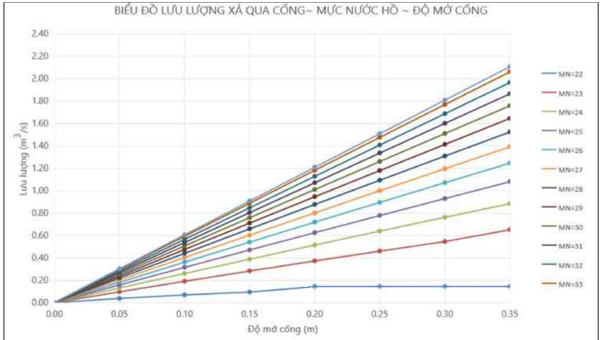
Hình PL6.1 Hình vẽ quan hệ mực nước hồ ~ Q xả cống ~ Độ mở cống lấy nước
