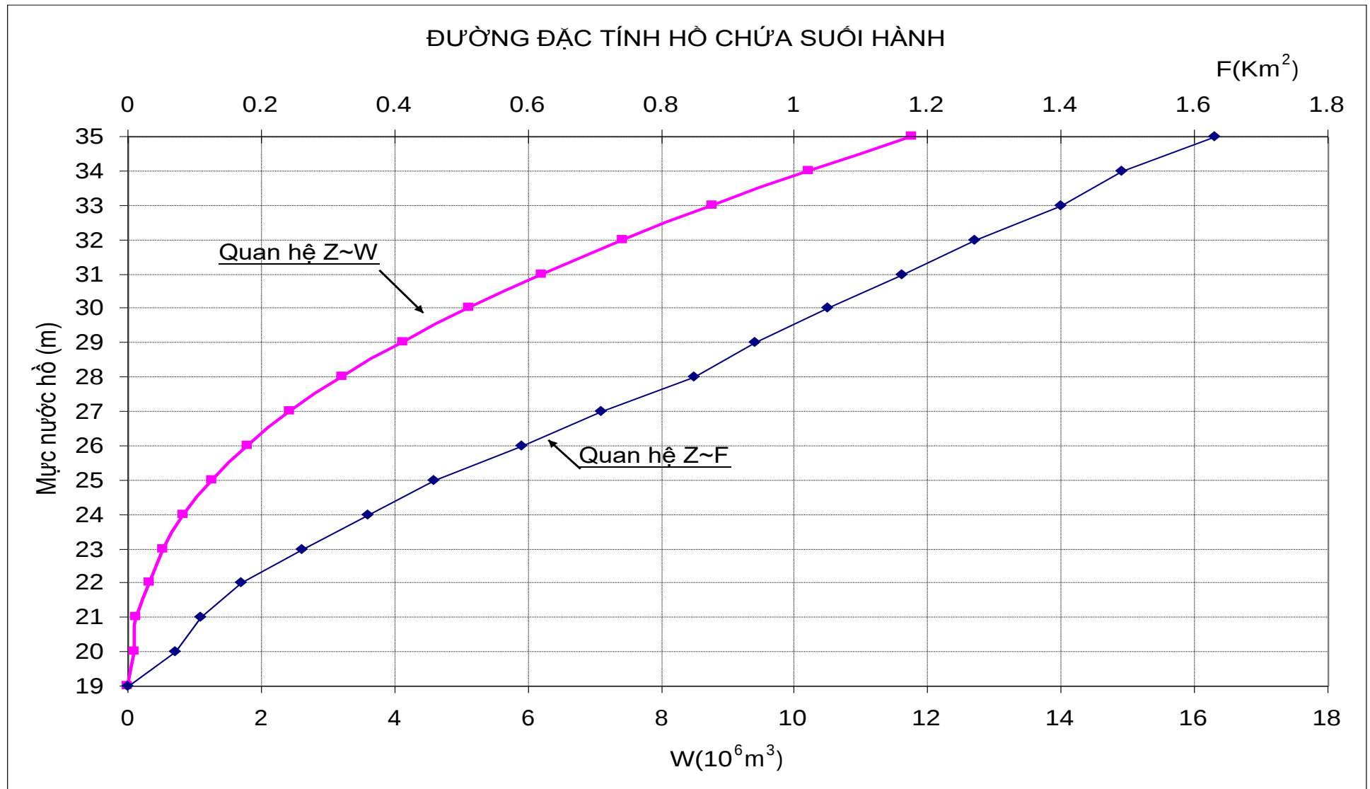
Hình PL8.1 Đường đặc tính hồ chứa nước Suối Hành
