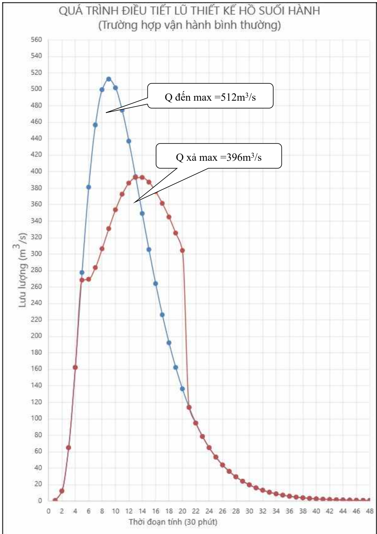
Hình PL 4.1: Quá trình điều tiết lũ thiết kế hồ suối hành
