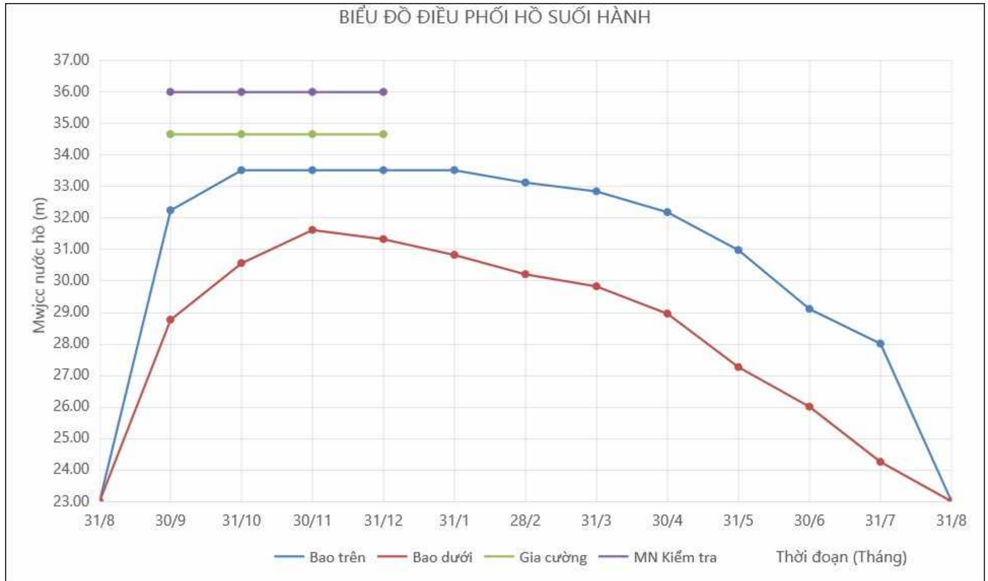
Hình PL7.1 Biểu đồ điều phối hồ chứa nước Suối Hành
